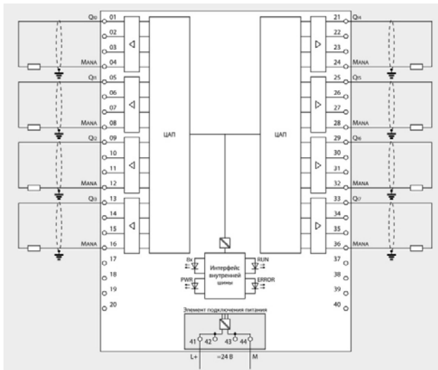
Формирование сигналов силы тока
