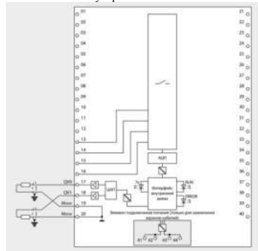
С управляющими сигналами напряжения
