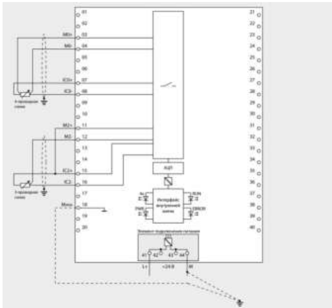
Подключение термометров сопротивления
