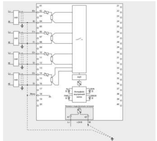
4-проводное подключение датчиков силы тока
