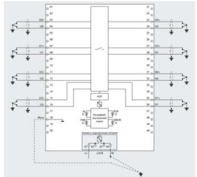
Подключение заземленных термопар
