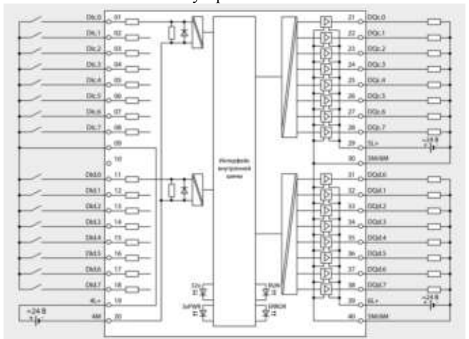
Соединитель X12 (только в CPU 1512C-1 PN)
