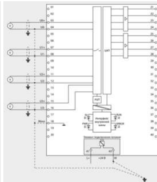
Подключение датчиков напряжения
