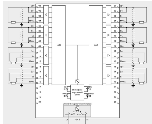
Формирование сигналов напряжения
