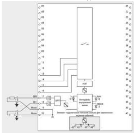
С управляющими сигналами силы тока
