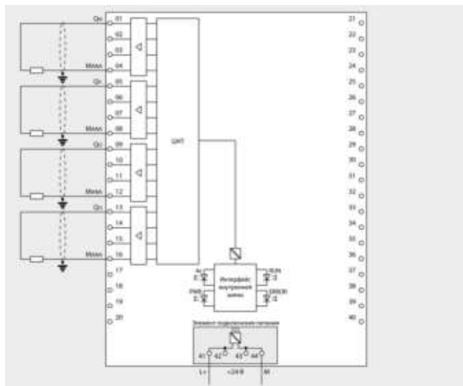
Формирование сигналов силы тока
