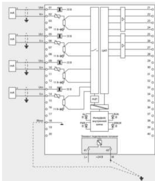
2-проводное подключение датчиков силы тока
