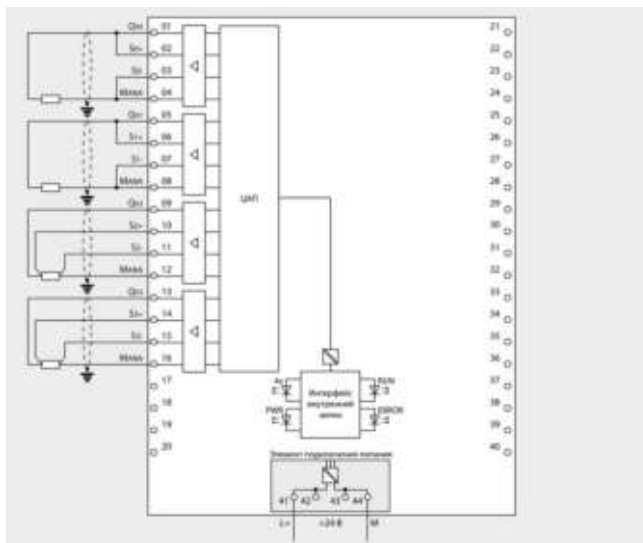
Формирование сигналов напряжения
