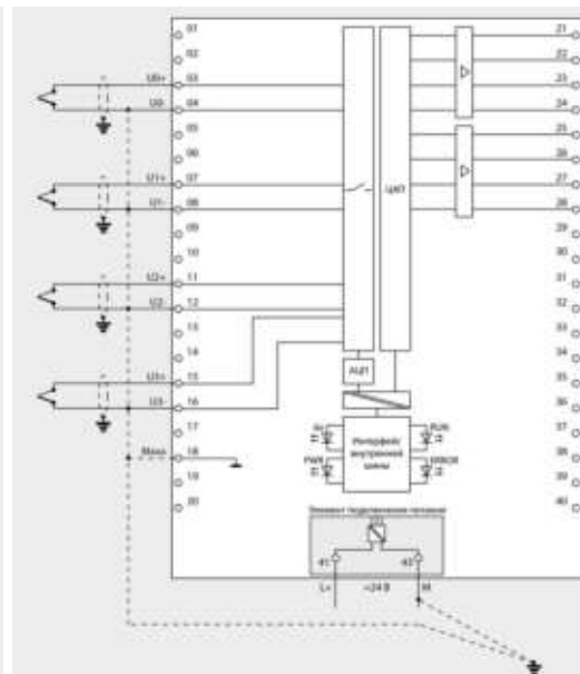
Измерение температуры с помощью термопар, внутренняя компенсация
