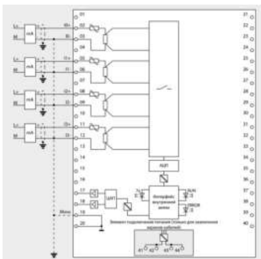
Подключение датчиков силы тока
