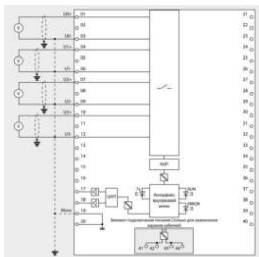
Подключение датчиков напряжения
