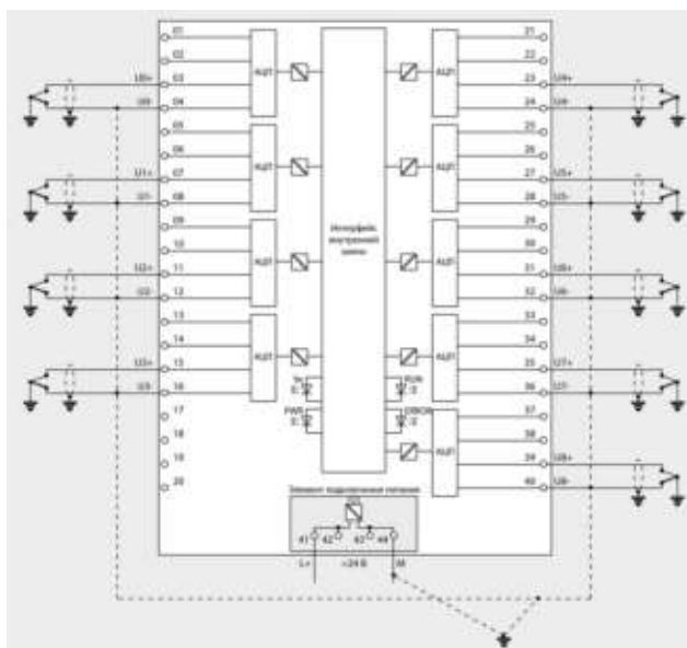
Подключение заземленных термопар
