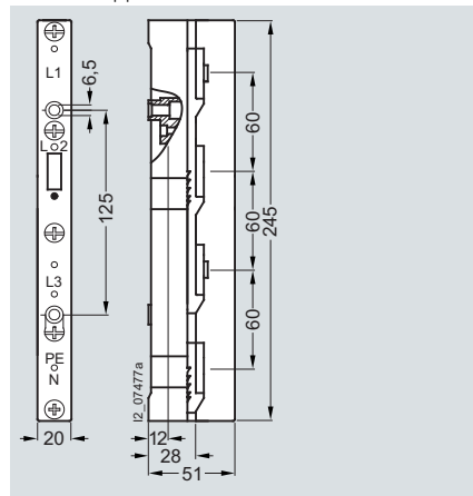
8US19 23-4AA00
