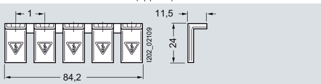
5ST3 655-0HG
