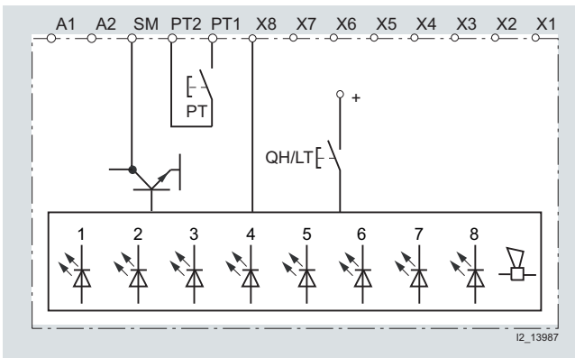
7LQ3 356, 7LQ3 357
