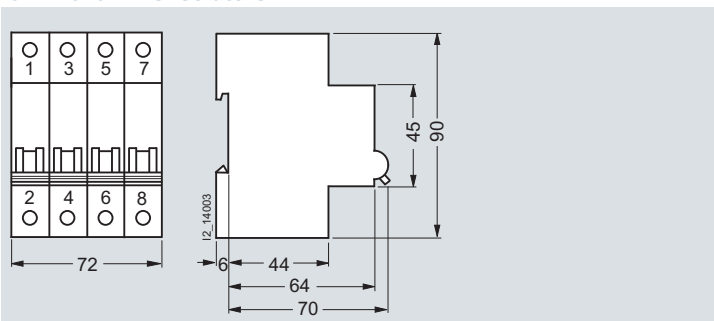
5TE2 515-1
