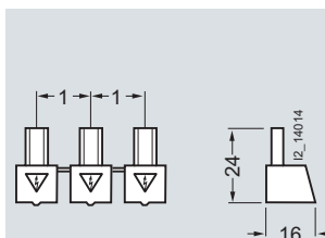
5ST3 666-1HG
