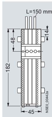
8US12 51-5DM07
