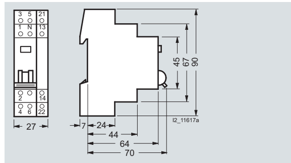
5TE8 118 5TE8 218
