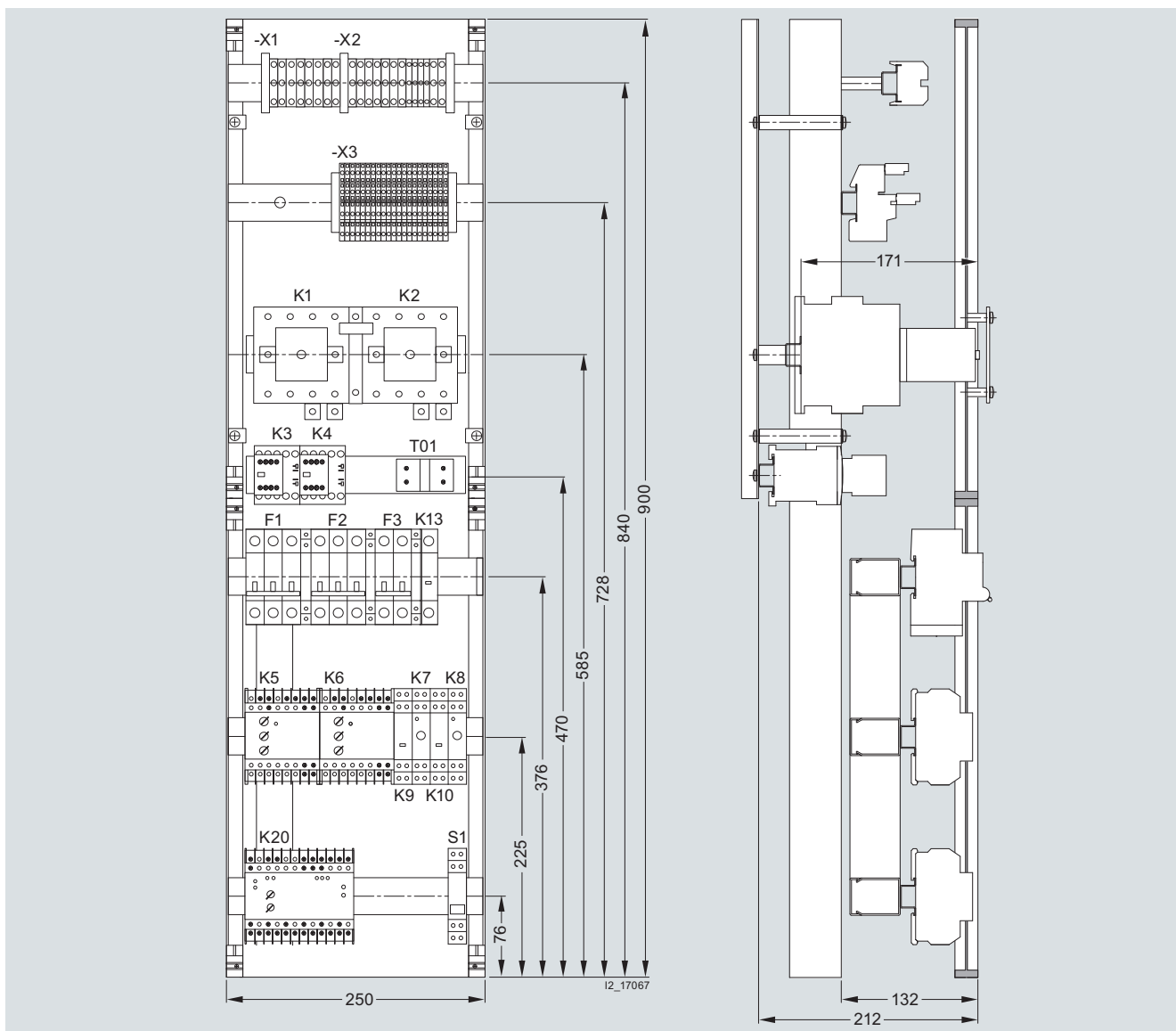
7LQ3 362
