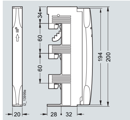
5SH5 538
