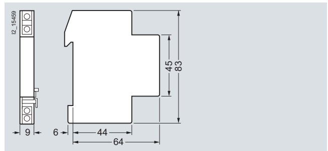
3NW7 903
