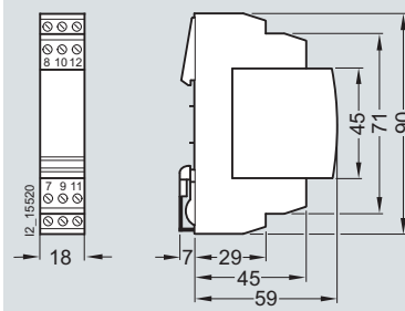
5SD7 5..
