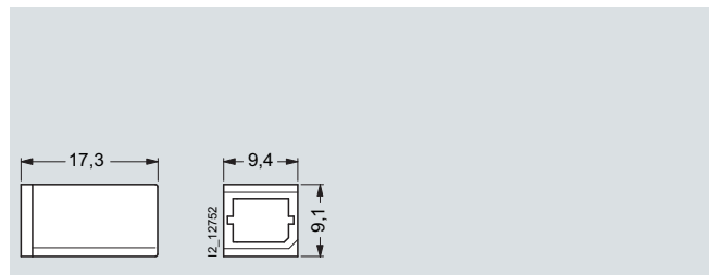
7LF4 940-1, 7LF4 940-2
