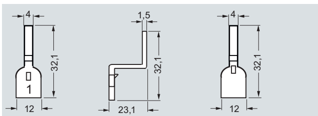
5ST3 512-0
