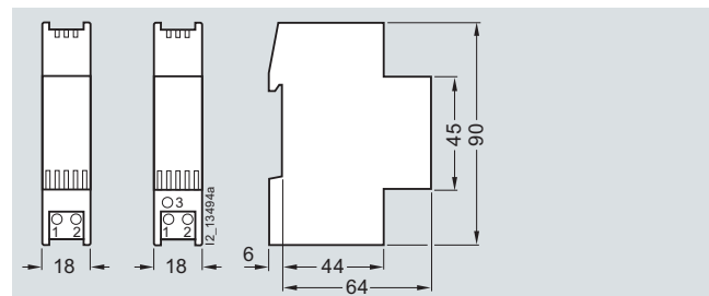
7LQ2 204 7LQ2 205
