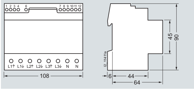
7KT1 3.0
