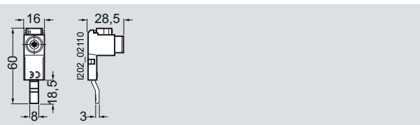
5ST3 770-0HG
