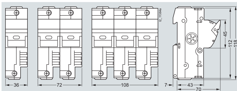
3NC1 29.
