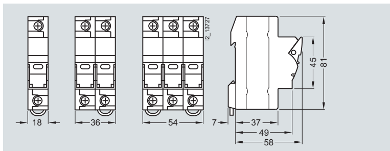
3NW7 5.3-0HG
