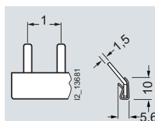
5ST3 763 5ST3 765
