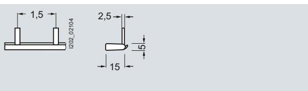
5ST3 701-2HG
