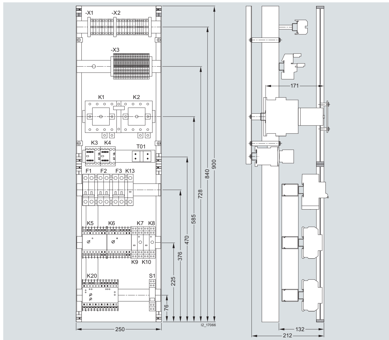
7LQ3 361
