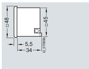
7KT5 5
