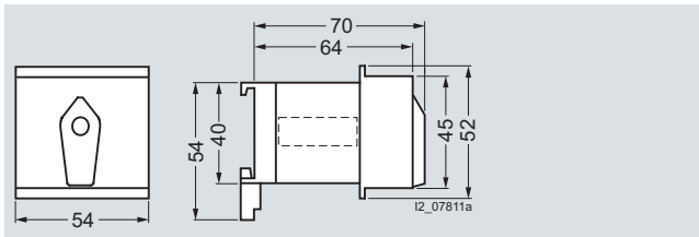
7KT9 010 7KT9 011
