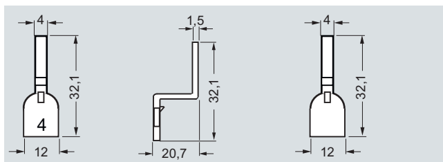
5ST3 515-0
