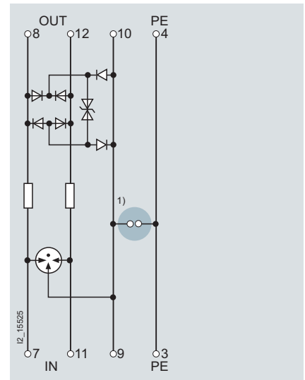
5SD7 530-3
