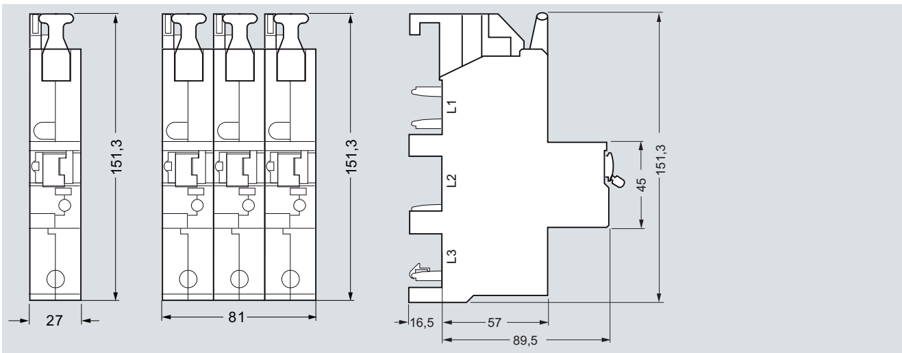
5SP3 7...-2 1P
