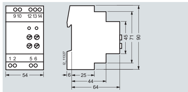
7LQ2 101 7LQ2 103
