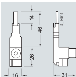
5ST3 666-0HG
