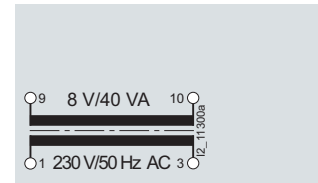
4AC3 540
