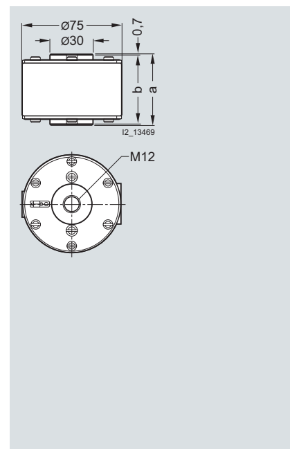
3NC3 4...-6
