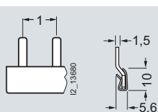
5ST3 762 5ST3 764
