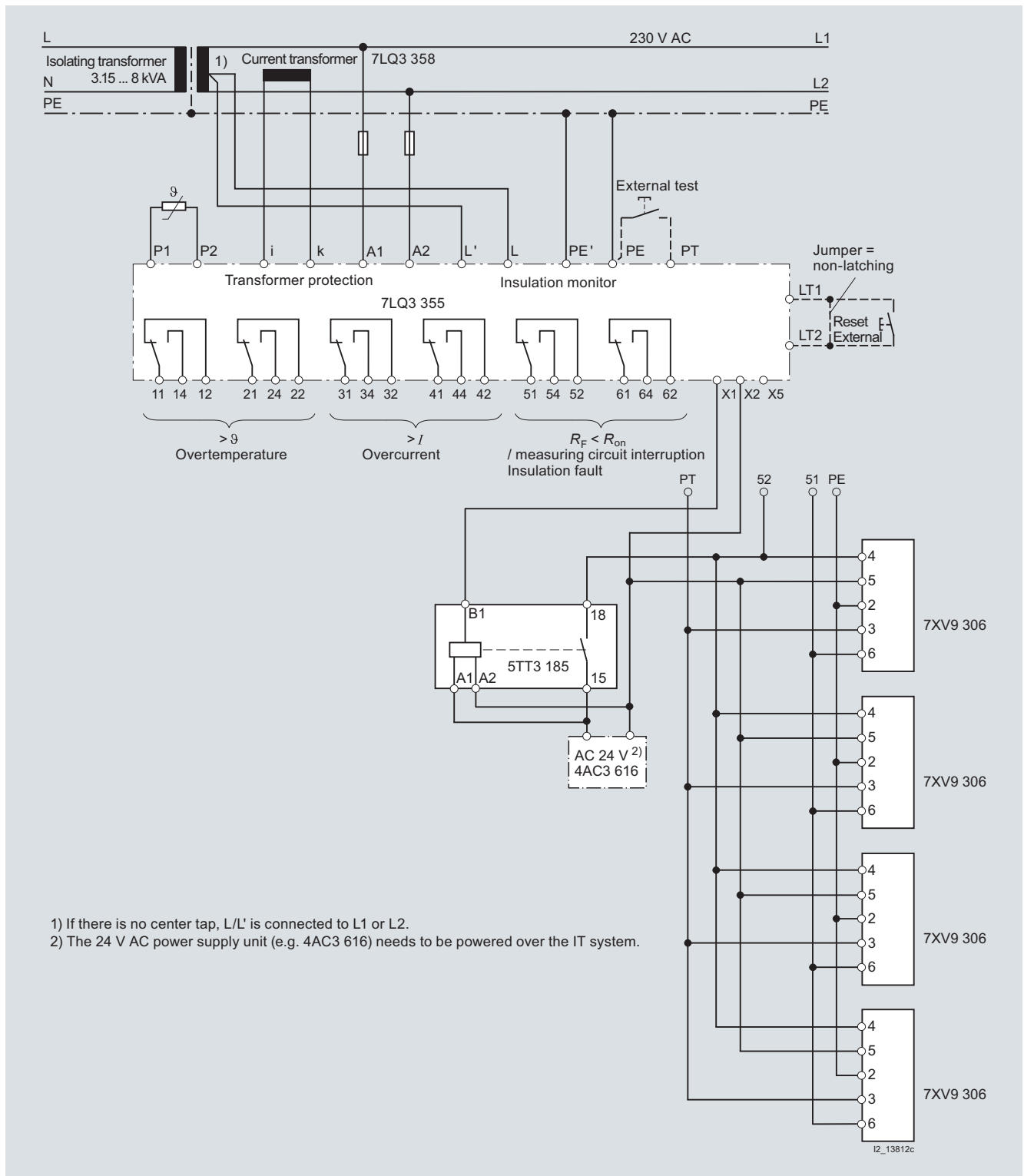
7LQ3 355
