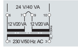
4AC3 640
