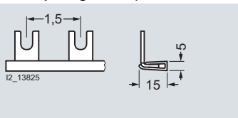
5SH5 517
