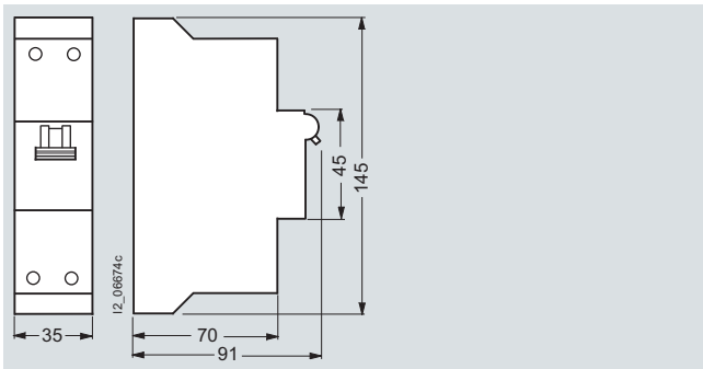
5SP3 7..., 5SP3 7...-1
