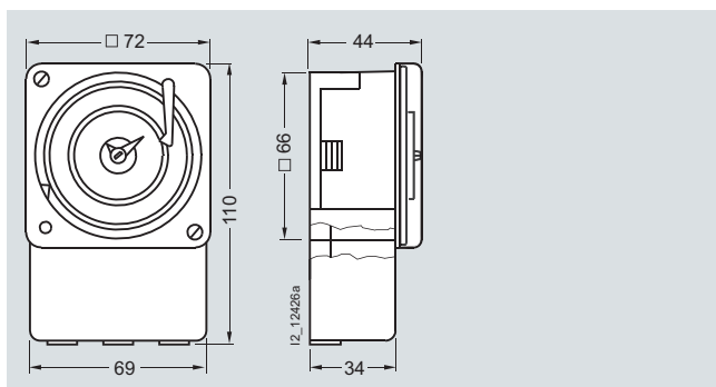
7LF5 301-0 7LF5 305-0
