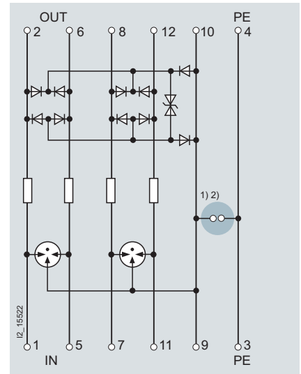
5SD7 550-4
