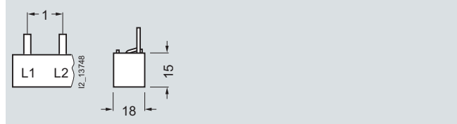
5ST3 704 5ST3 705
