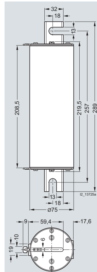
3NE9 6...-1C
