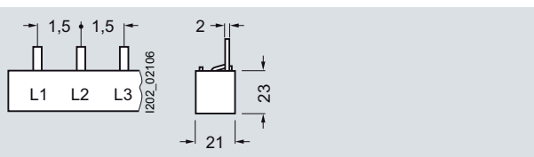
5ST3 710-2HG
