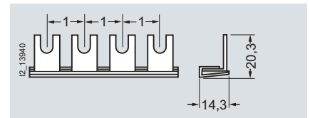
5SD7 490-4
