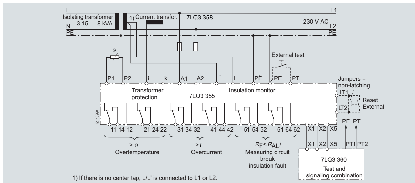
7LQ3 355
