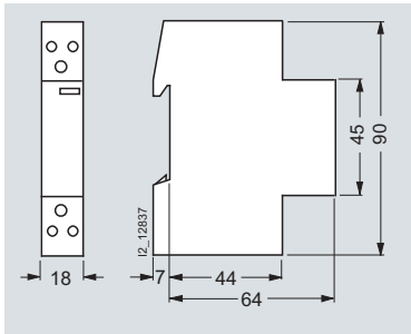
5TT5 80.-0 5TT5 80.-2
