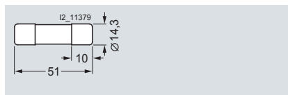
3NC1 4..
