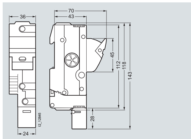
3NC1 291-5
