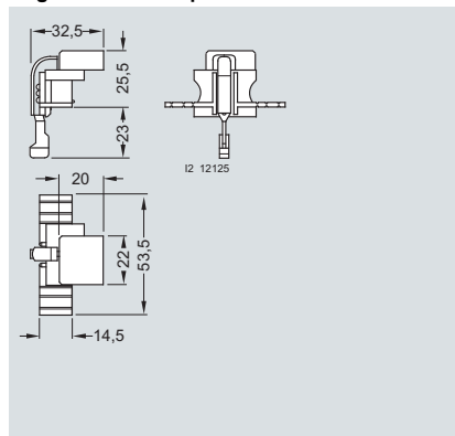
3NX1 024
