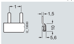
5ST3 762 5ST3 764
