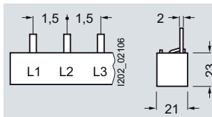
5ST3 710-2HG
