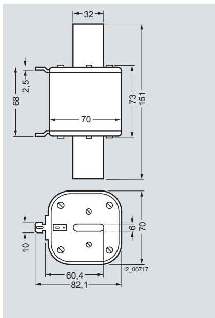
3NE1 43...-0, 3NE1 43...-1
