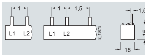
5ST3 704 5ST3 706 5ST3 705 5ST3 707 5ST3 734 5ST3 736 5ST3 735 5ST3 737 Two-phase
