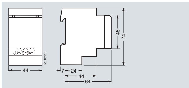
5TE6 801
