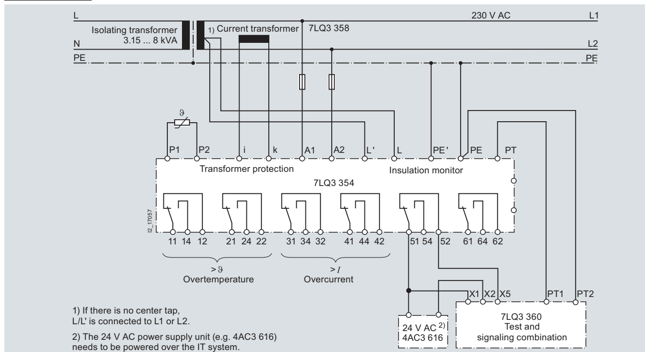
7LQ3 354
