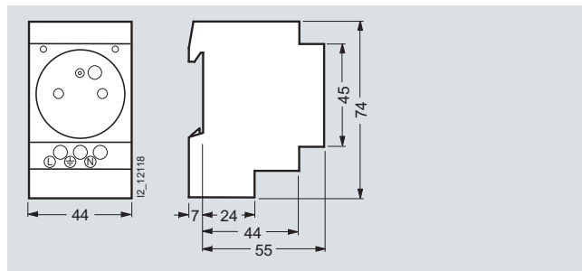
5TE6 803
