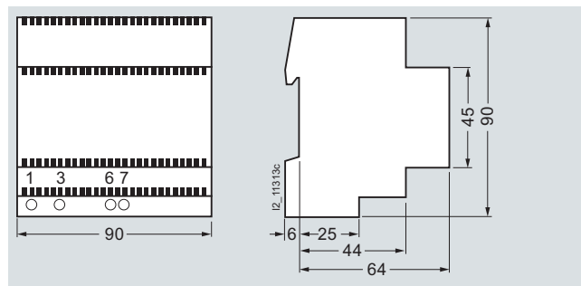
4AC2 401
