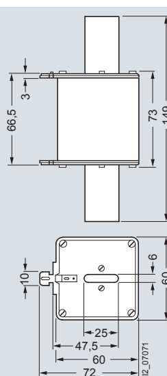
3NE1 33...-0, 3NE1 33...-2
