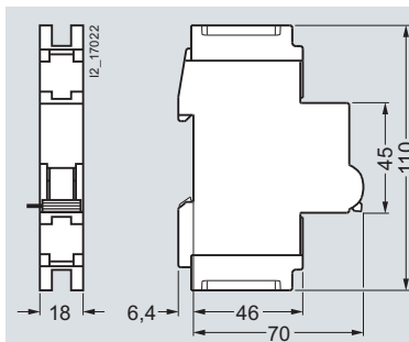
5ST3 030-0HG 5ST3 031-0HG
