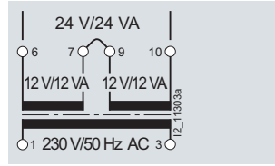
4AC3 624
