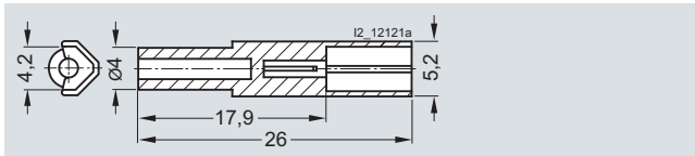
2P, 125 A
