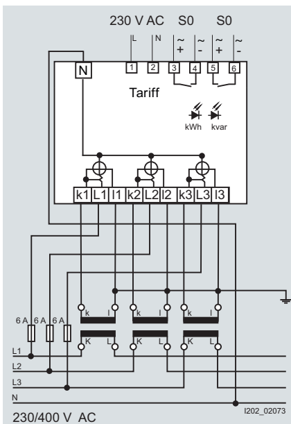
7KT1 540
