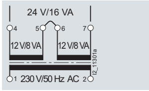
4AC3 616
