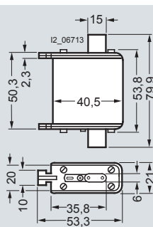
3NE1 8...-0
