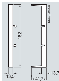
8US19 98-2BM00
