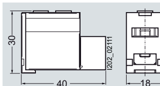
5ST3 770-1HG
