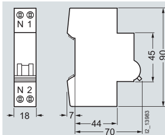
1P+N N pole left
