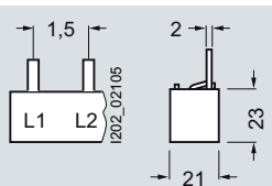
5ST3 705-2HG
