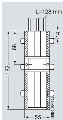
8US12 61-5FM08
