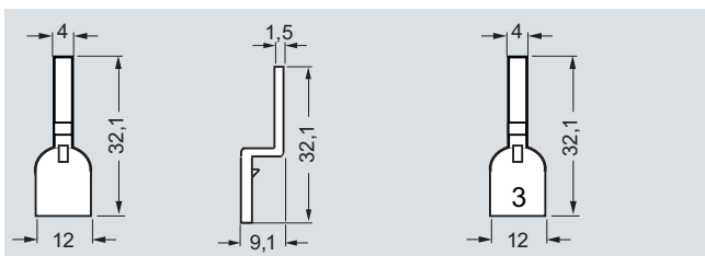
5ST3 514-0
