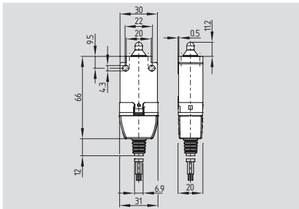
Z/T 196-.. L1
