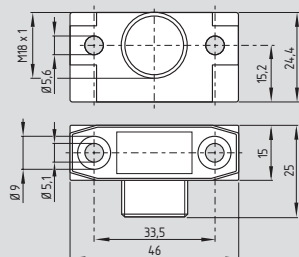
Actuator CST 180-1
