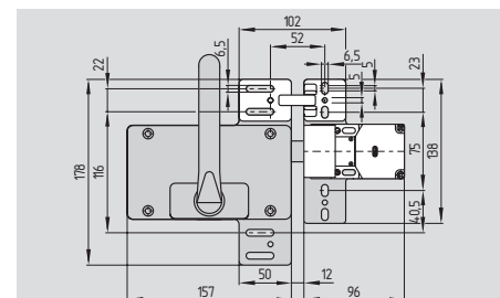
Actuator AZ 16-STS30
