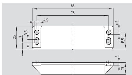
BPS 33
