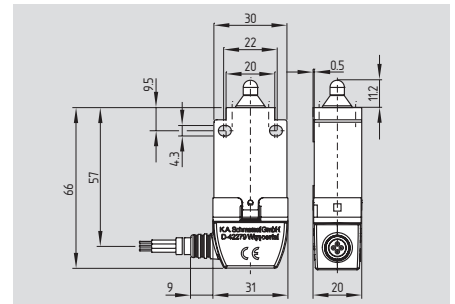
Z/T 196-.. L3
