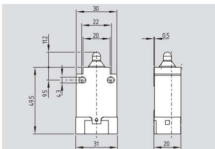
Z/T 196-..
