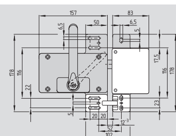
AZ 415-STS30
