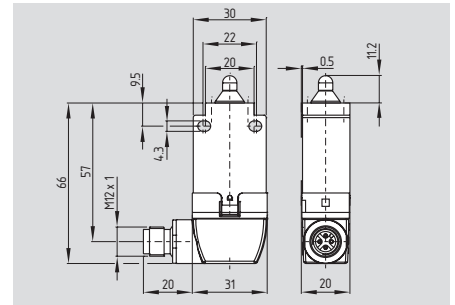
Z/T 196-.. ST3
