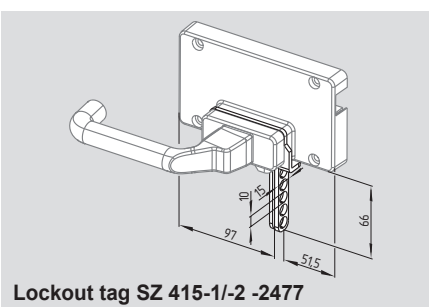
Lockout tag SZ 415-1/-2
