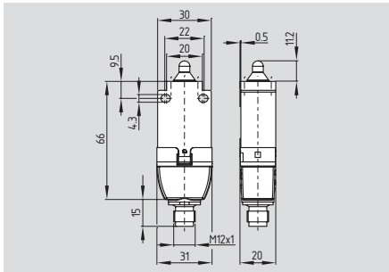
Z/T 196-.. ST1
