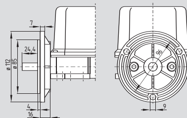
Flange FL1
