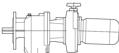
Stirnrad - Verstellgetriebemotor mit Reibradverstelleinheit Flanschausführung
