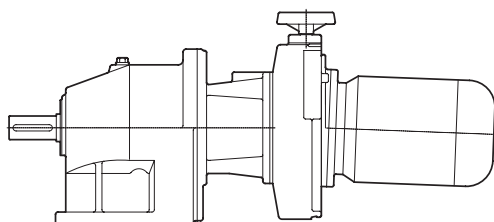
Stirnrad - Verstellgetriebemotor mit Reibradverstelleinheit Fussausführung
