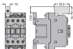
Клеммы увеличенного размера G231 - 1 полюс
