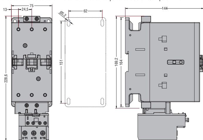
BF85 00E... - BF95 00E... - BF115 00E... - BF150 00E... трехполюсные с тепловым реле RF110
