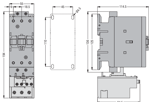
BF40 00E... - BF50 00E... - BF65 00E... - BF80 00E... трехполюсные с тепловым реле RF82
