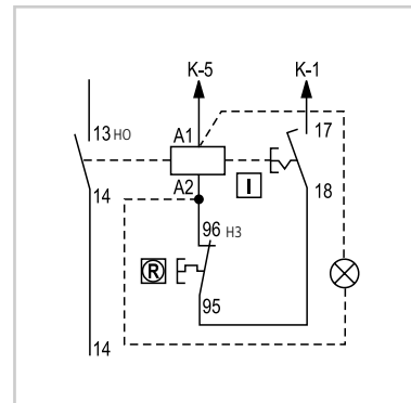
Цепь управления
