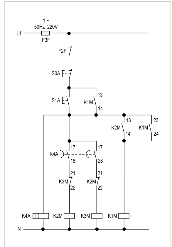
Цепь управления
