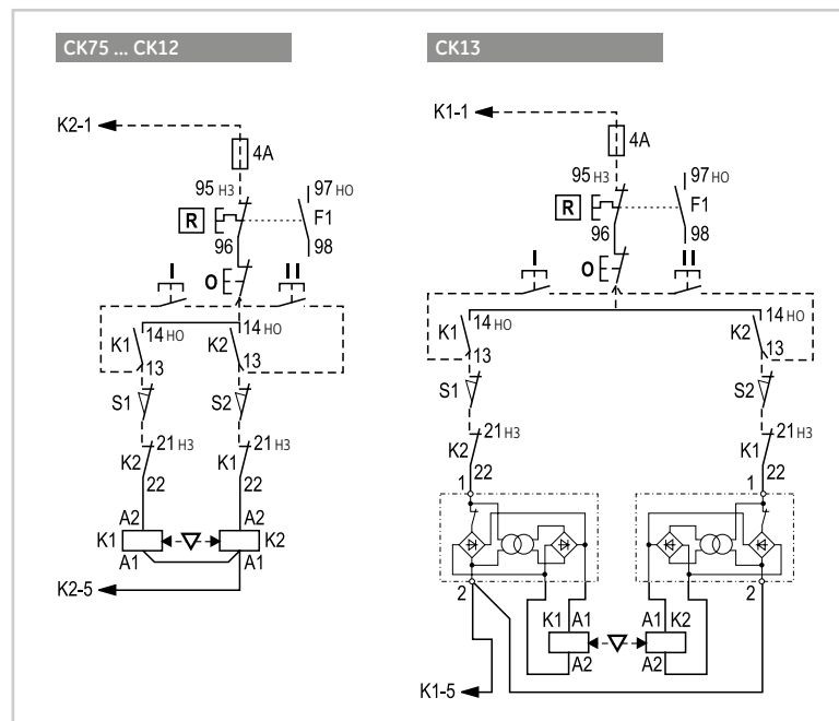
Цепь управления
