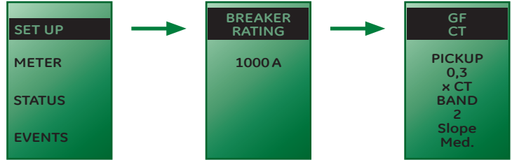
4-х проводная система
